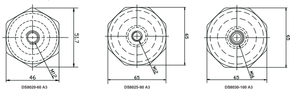
Profile 剖面图
