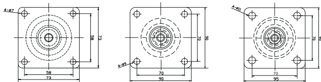
Profile 剖面图
